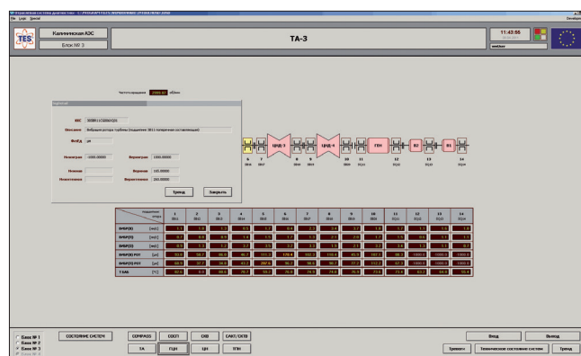
Obrazovka se záznamy vibrací rotoru
