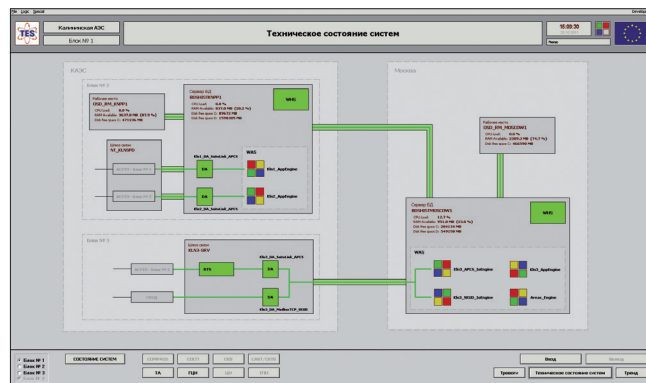
Obrazovka s technologickým uspořádáním systému
